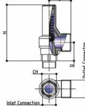
SCARICO CONVOGLIATO PIPED OUTLET
