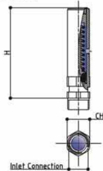
SCARICO LIBERO FREE OUTLET
